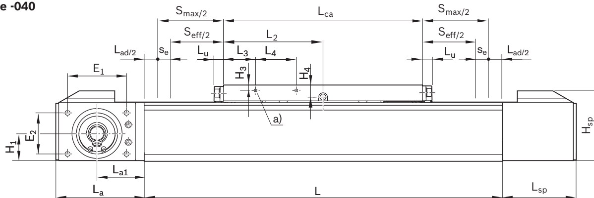
Size -040
