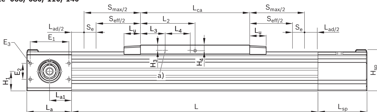
Size -065/-080/-110/-140
